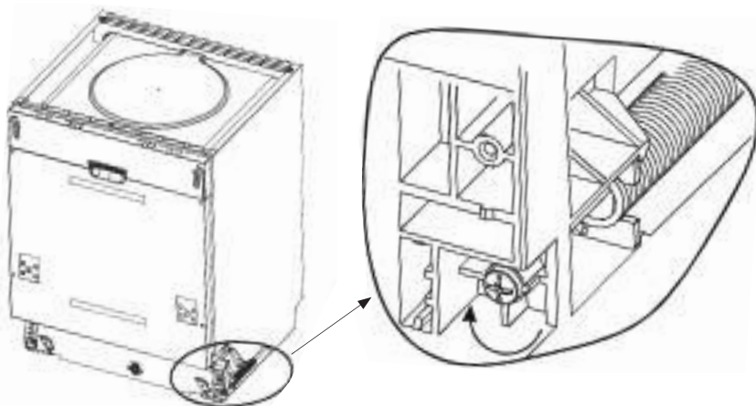
Рис. 6 Регулировка натяжения пружины дверцы посудомоечной машины
